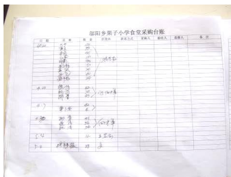
图 28 采购台账图
